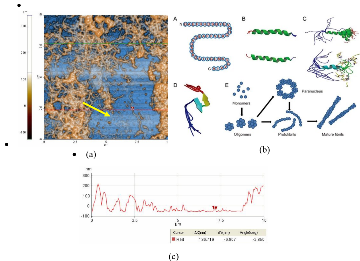
F(a) Imagine AFM bidimensionala, prezentata in mod “contrast imbunatatit”, scanata pe o suprafata de (10 \times 10) \mu\text{m}^2 ; (b) Structuri ale monomerului \beta A , fibrilelor și oligomerilor; (c) Detalii la scala nanometrica a liniei de profil indicate printr-o linie rosie in Fig. 8(a)
